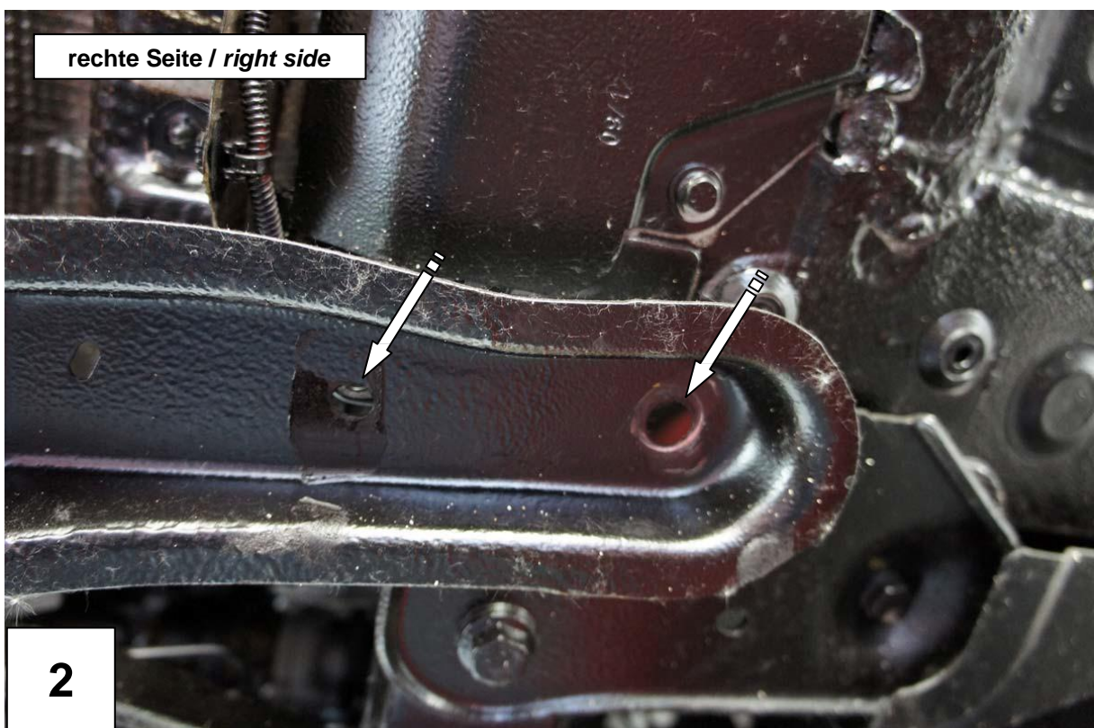
Befestigungspunkte Konsole B – rechts / Fixing points bracket B – right side
