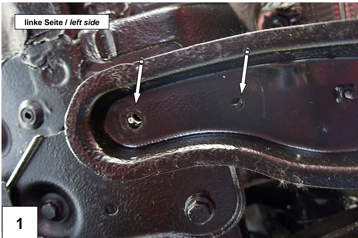
Befestigungspunkte Konsole B – links / Fixing points bracket B – left side
