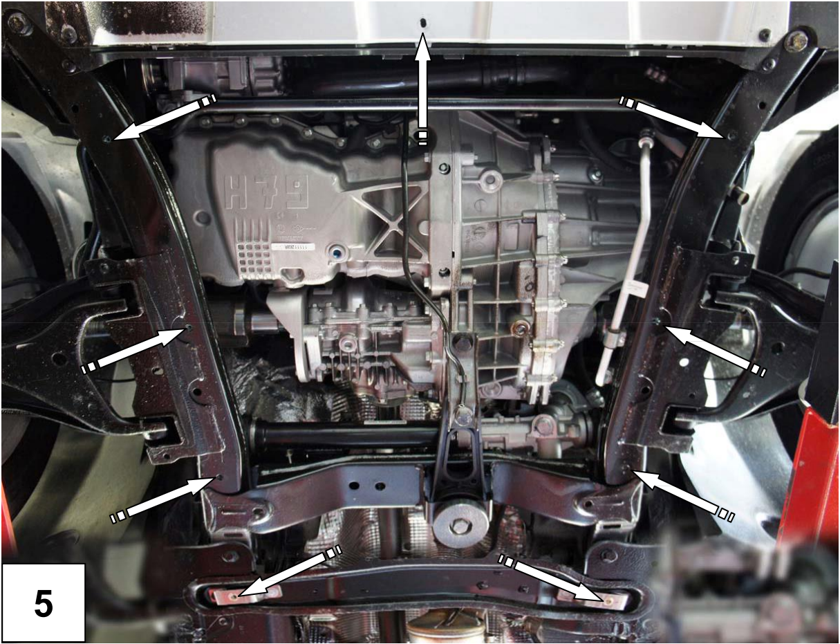
Befestigungspunkte Schutzplatte / Fixing points skidplate
