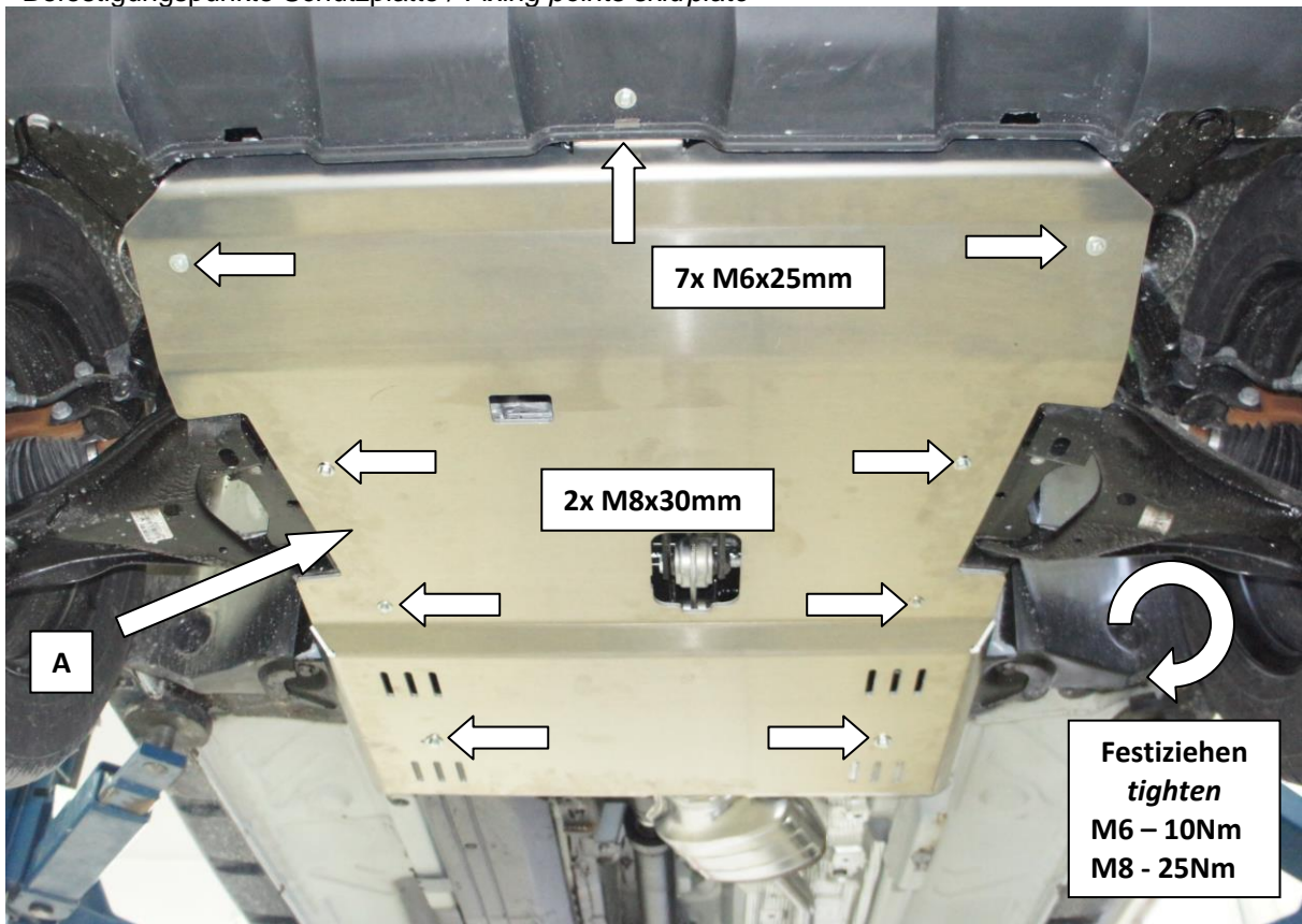
Schutzplatte anbringen / Attach skidplate
